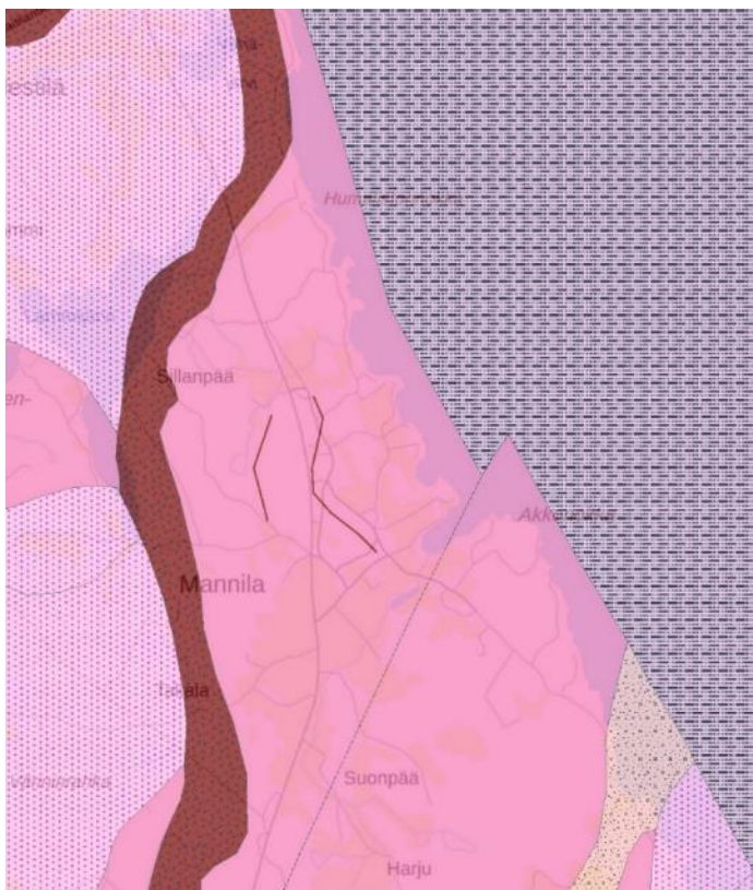
Kuva 4. Selvitysalueen kallioperä.
